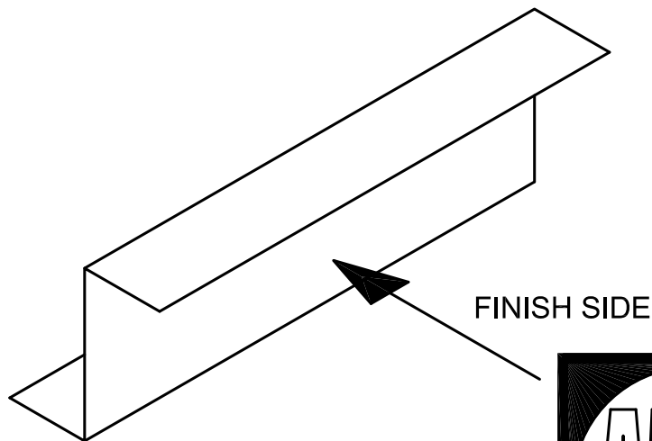
ISO VIEW N.T.S.
